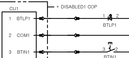
WCOP30-N B'd (DISABLED1 COP)
