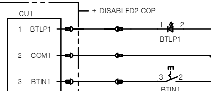
WCOP30-N B'd (DISABLED2 COP)
