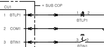
COP30D-N B'd (SUB COP)
